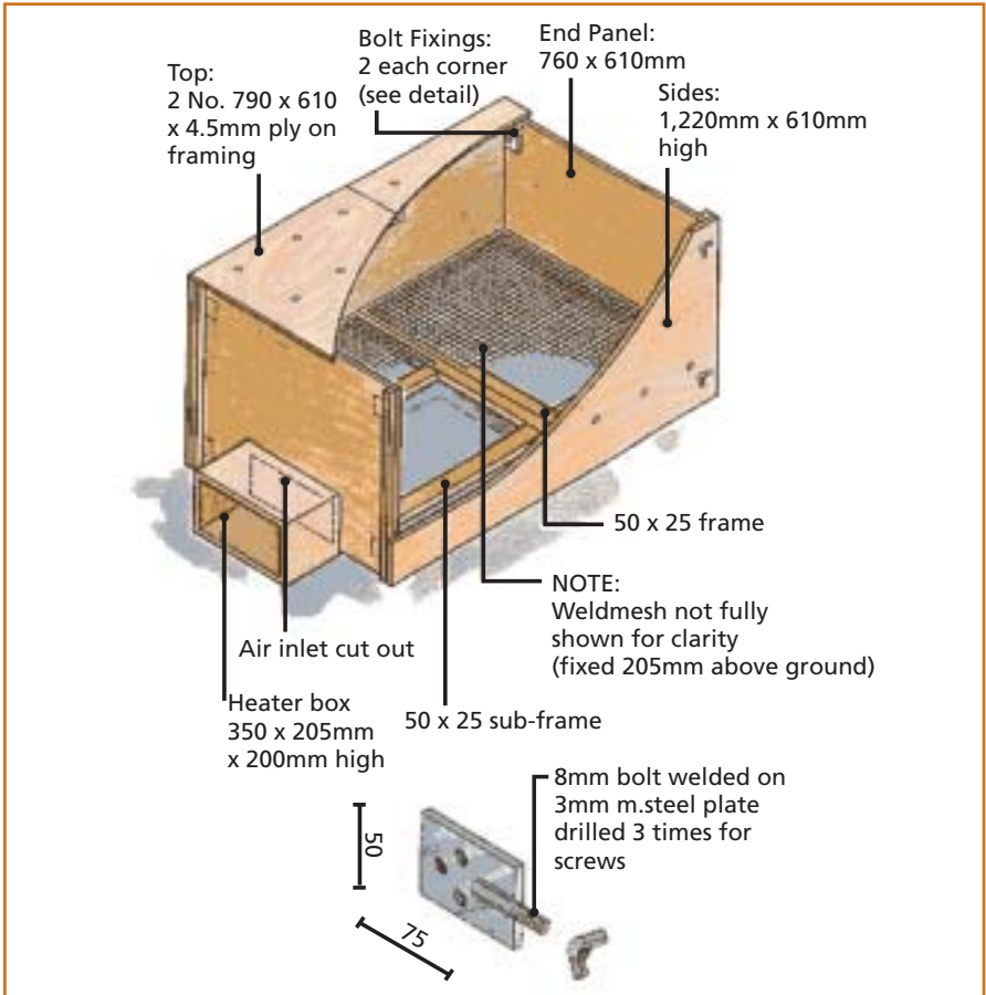
Lamb warming box.
